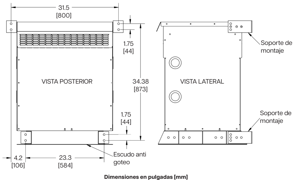
Dimensiones de montaje en pared DW3
